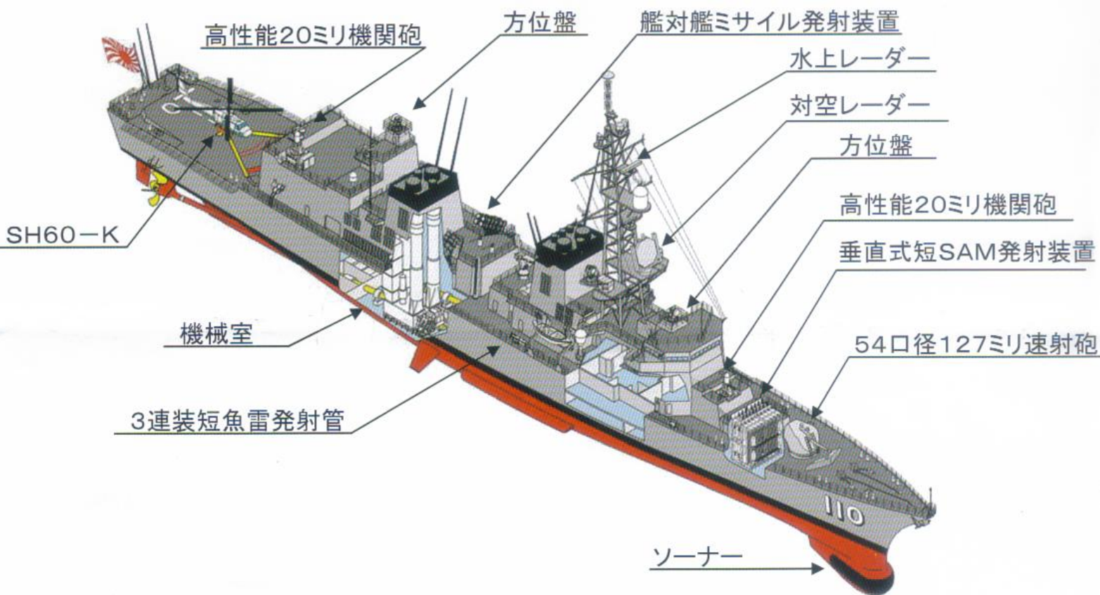
艦対艦ミサイル発射装置 (SSM-1B / Harpoon) 水上目標に対処するため、国産のSSM-1Bを発射する装置です。
